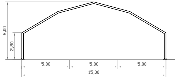
CORTE TRANSVERSAL
