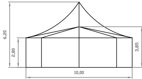
CORTE TRANSVERSAL
