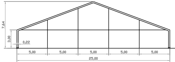
CORTE TRANSVERSAL
