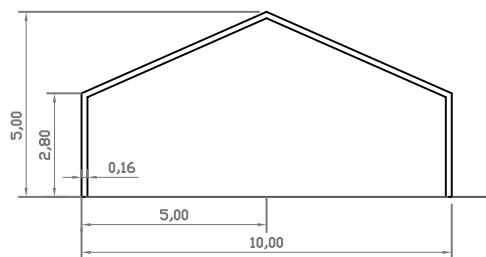
CORTE TRANSVERSAL
