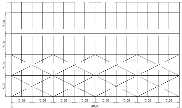
PLANTA
