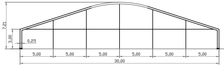
CORTE TRANSVERSAL
