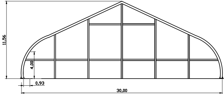
CORTE TRANSVERSAL
