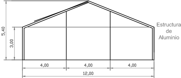
CORTE TRANSVERSAL
