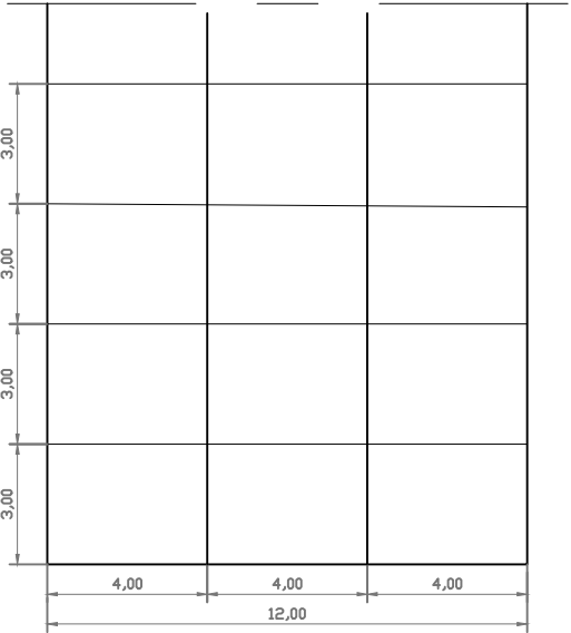
PLANTA
