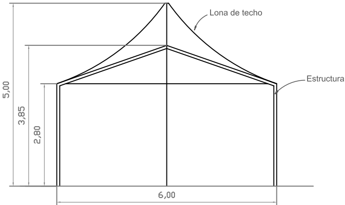
CORTE TRANSVERSAL
