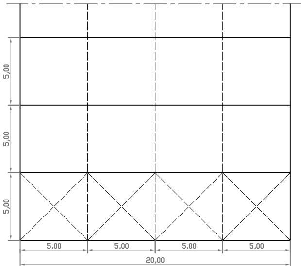
PLANTA
