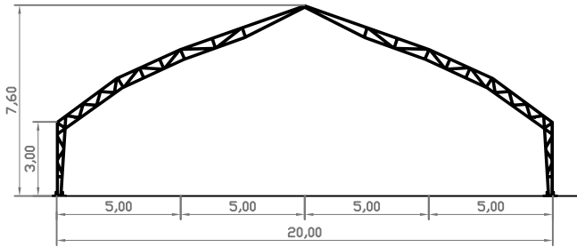
CORTE TRANSVERSAL
