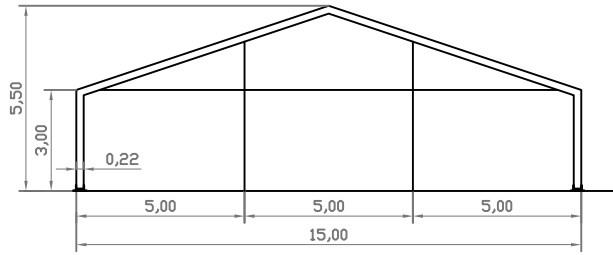
CORTE TRANSVERSAL
