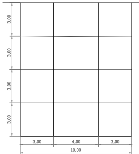
PLANTA
