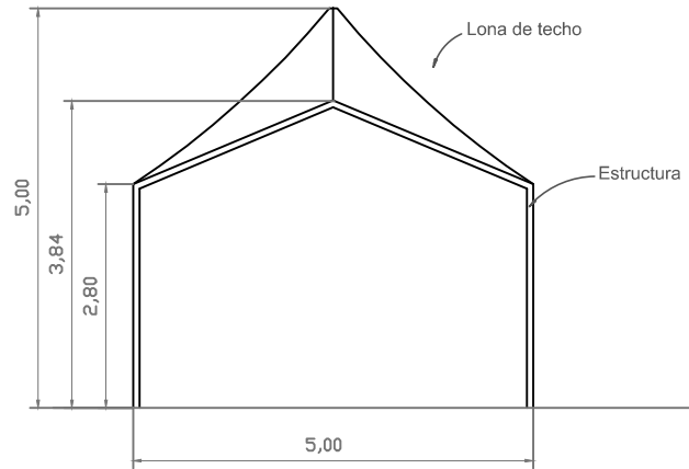
CORTE TRANSVERSAL
